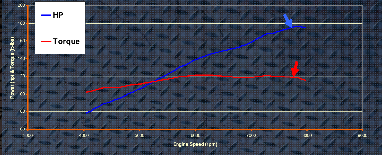
Z1 Turbo Power Test
